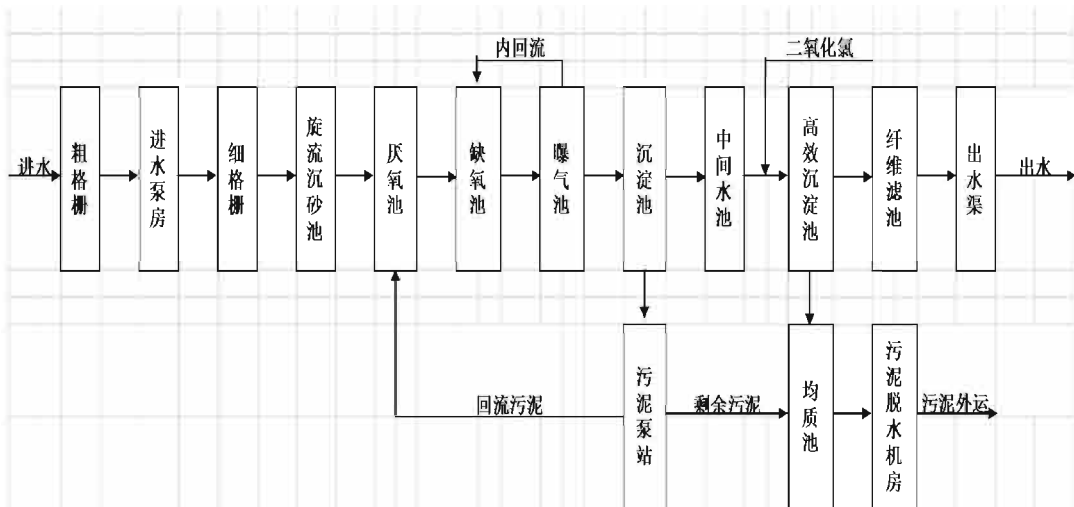
图 5-3 A2/O 工艺流程图
