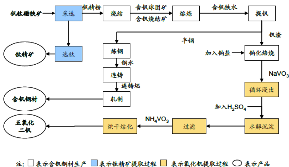
图 9-2 发行人钒钛产品及含钒合金钢的生产流程
