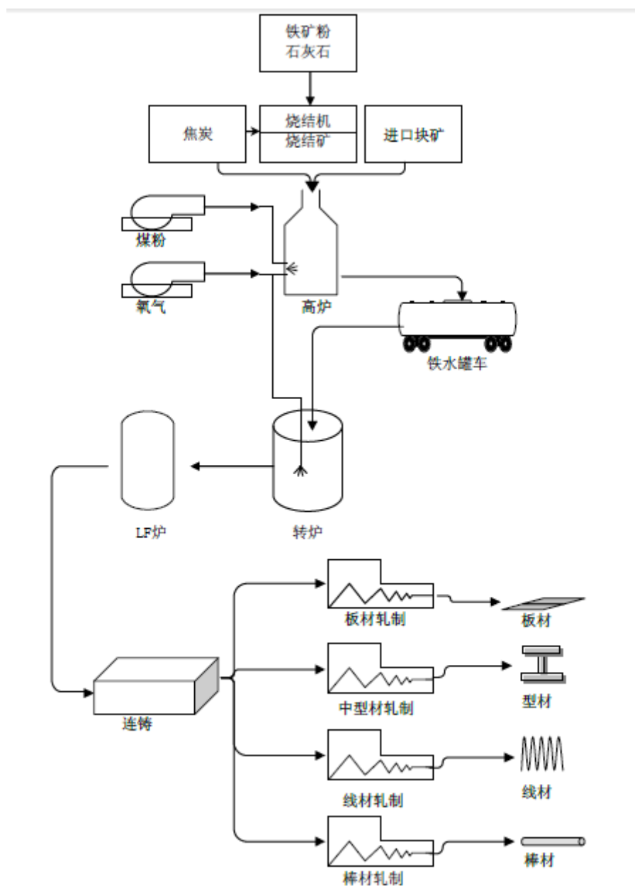
图 9-1 发行人钢铁产品工艺流程
