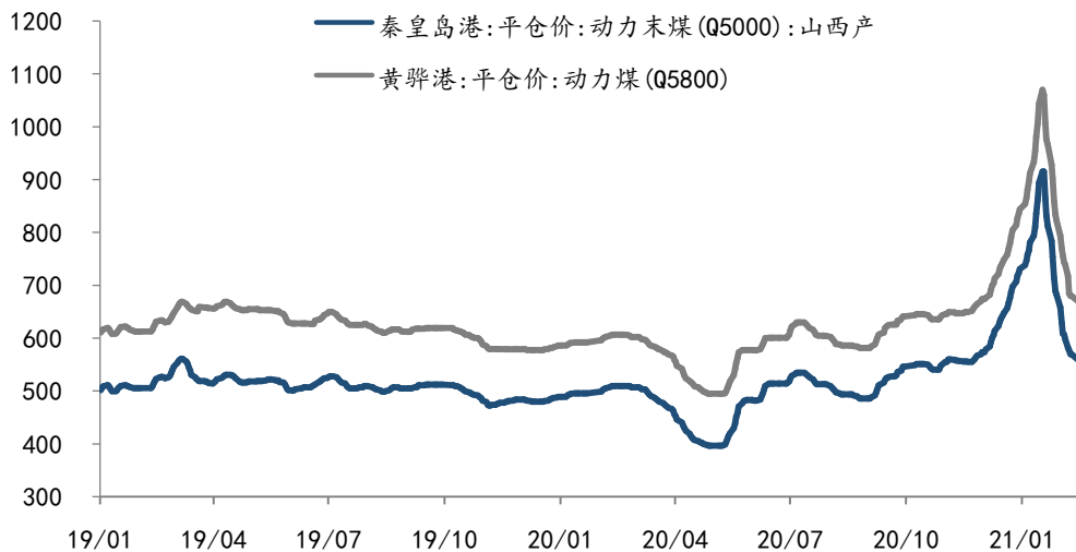
图表 1：动力煤价格持续下跌（元/吨）
